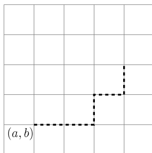
Figure 1: The path p = EENEN .
